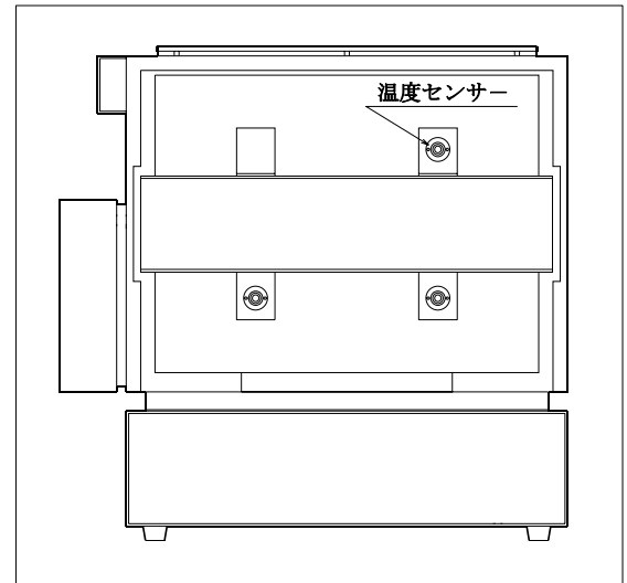
《後部パネルを取り外し時の後面図》
